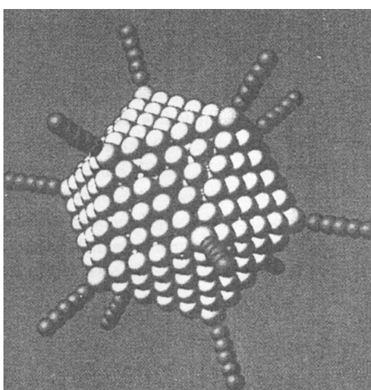
2 Modell des sphärischen (ikosaedrischen) Adeno-Virus (s. z.B. Peter Sitte, Anm. 5)
