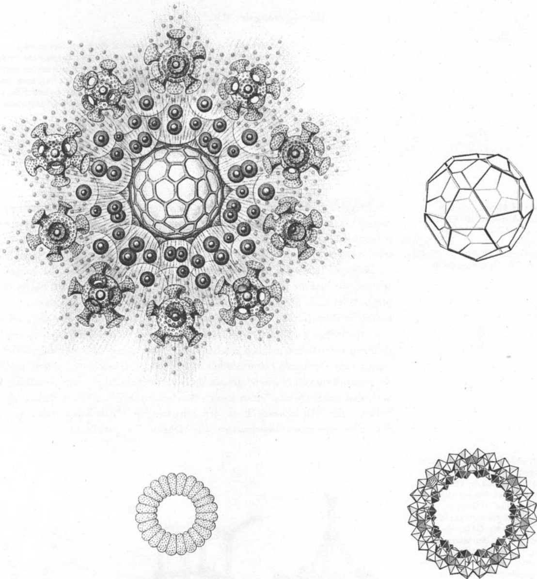
3 Kugel- und kreisförmige Gebilde: Zwei Polycyttaria/Vereins- Strahlige (◊Soziale Radiolarien◊) aus Ernst Haeckels Buch Kunst- Formen der Natur (Tafel 51, links) und Modelle von strukturell ver- gleichbaren in Bielefeld synthe- tisierten Riesenmolekülen, die im Aufsatz behandelt werden (rechts).
