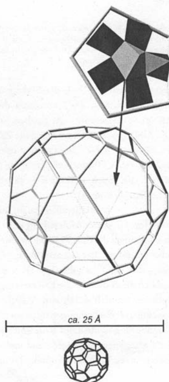
6 Kugel- bzw. Fußball-förmige Gebilde: Struktur des aus 60 Molybdänatomen bestehenden ikosaedrischen Mo_{60} -Fragmentes des genannten Superfullerens mit 12 regelmäßigen Fünfecken und 20 (trigonalen) Sechsecken. Eine strukturierte pentagonale Einheit ist in Polyederdarstellung separat abgebildet. Jede pentagonale Baueinheit besteht aus einer zentralen pentagonalen Bipyramide, die mit fünf Oktaedern über Kanten verknüpft ist. Die einzelnen Polyeder bestehen wiederum aus (sieben oder sechs) Sauerstoffatomen mit jeweils einem zentralen Metallatom (oben). Im gleichen Maßstab ist zum Vergleich das Fußballmolekül, das C_{60} -Fulleren, dargestellt (unten).
