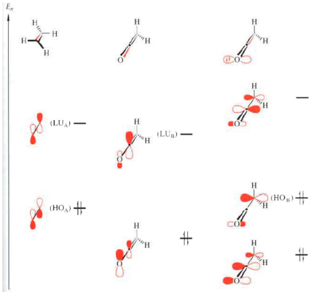
Grenzorbitale von Ethen und Keten
