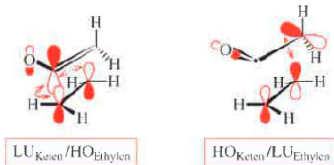
Grenzorbital-Wechselwirkungen bei der konzertierten [2+2]-Cycloaddition von Keten an Ethen
