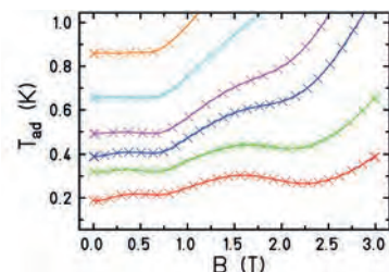
Kurven konstanter Entropie, auf denen sich das Molekül \{Gd_n\} abkühlt, wenn das Magnetfeld B verringert wird
