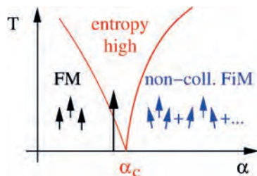
Quantenphasenübergang bei \alpha_c für das magnetische Molekül \{Fe_{10}Gd_{10}\}
