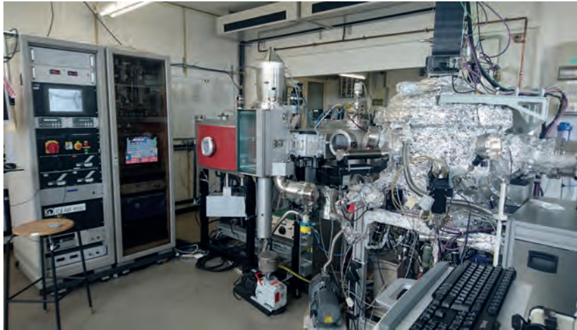
Kombinierte Sputter- und Molekularstrahlanlage der Arbeitsgruppe Reiss: mit dieser Anlage können dünne Schichten aus verschiedenen Materialien atomlagengenau hergestellt werden.
